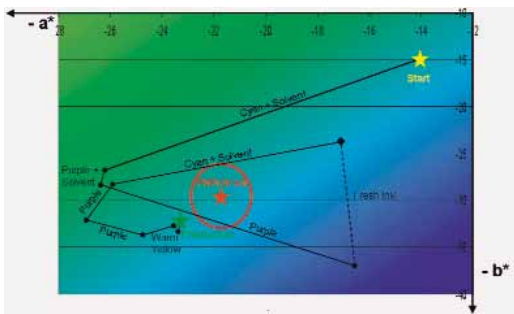
Az eredeti és a gépi mintán végzett spektralfotometriai mérés valós, jól használható értéket szolgáltat a színkorrekcióhoz
